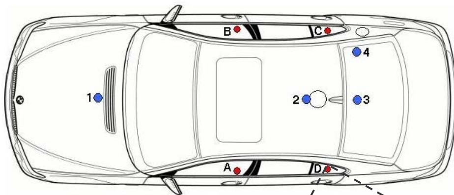
1-4: H 2 -Sensoren A-D: rot blinkende LEDs in den Türpins
