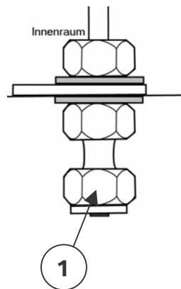
Aufbau Spülanschluss
